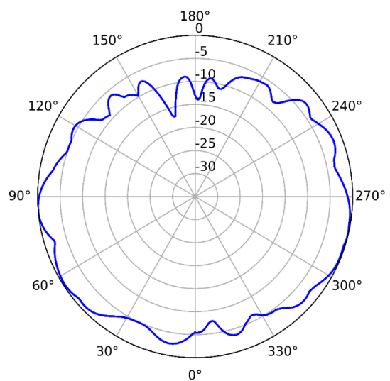
5GHz (Vertical)
